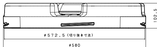
組正面図
