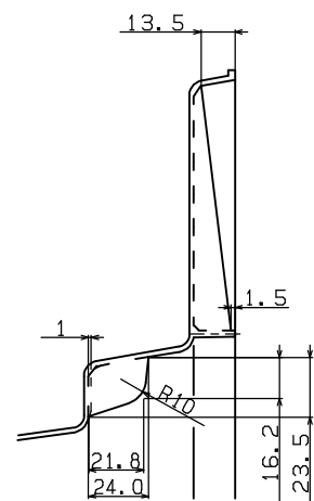
Sec A-A'
