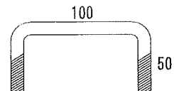
④取手 片ゲート両面 2ヶ
