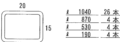
③クロス用材
